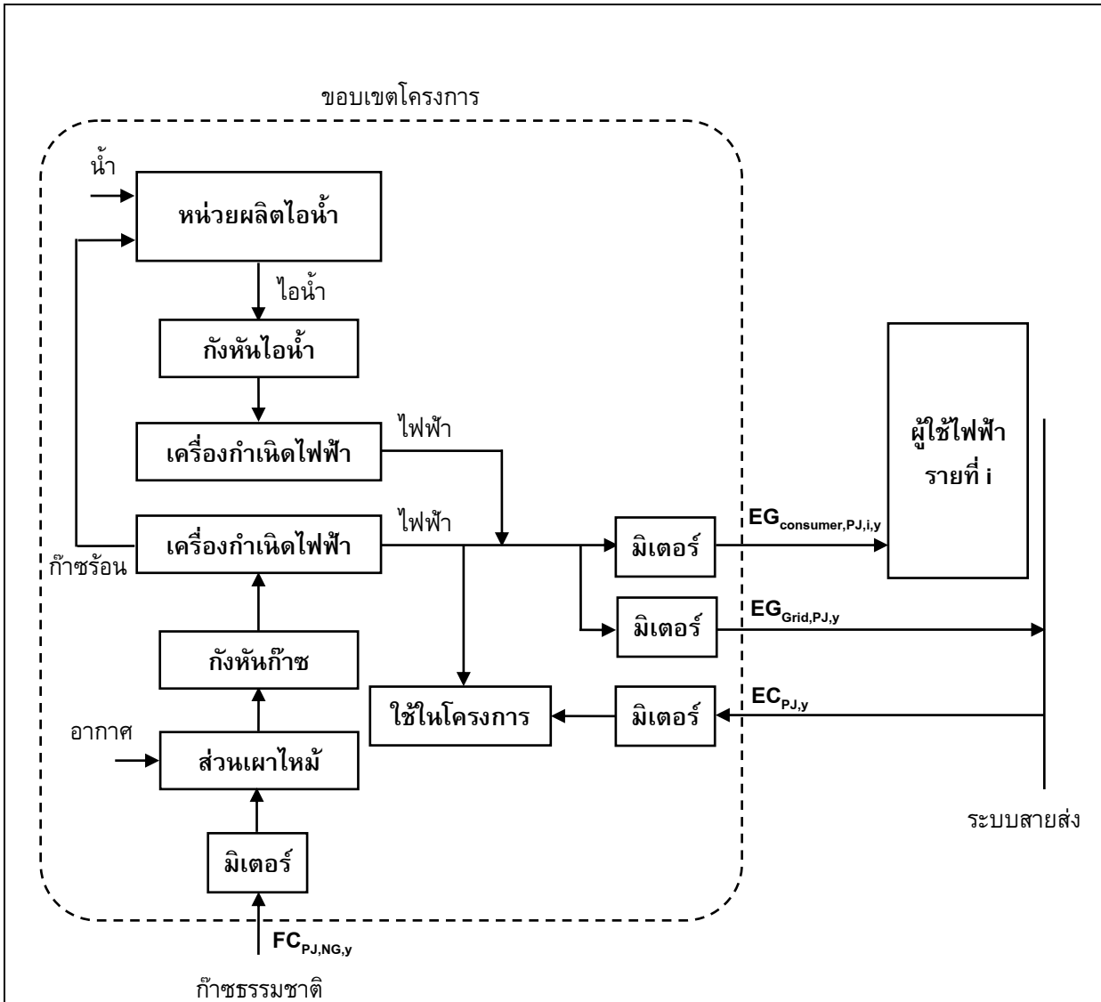
รูปที่ 2 ตัวอย่างแผนภาพแสดงพารามิเตอร์ที่ใช้ในการคำนวณกรณีโรงไฟฟ้าพลังความร้อนร่วม
