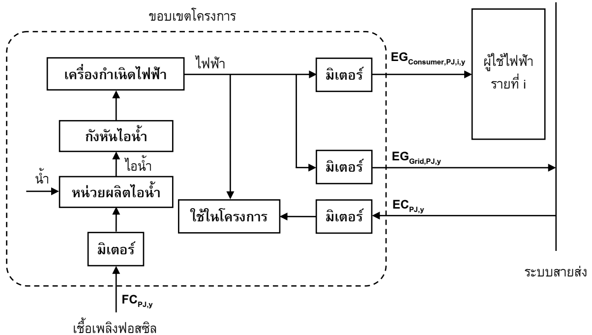
รูปที่ 1 ตัวอย่างแผนภาพแสดงพารามิเตอร์ที่ใช้ในการคำนวณกรณีโรงไฟฟ้าพลังความร้อน
